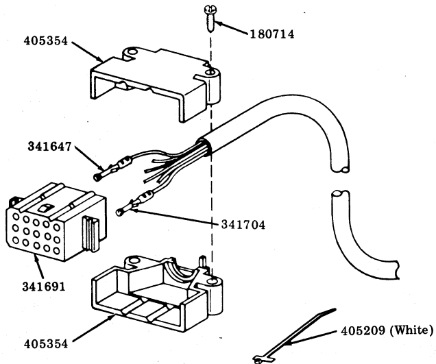
Fig. 15—405372 40KDA Stub Cable Assembly
