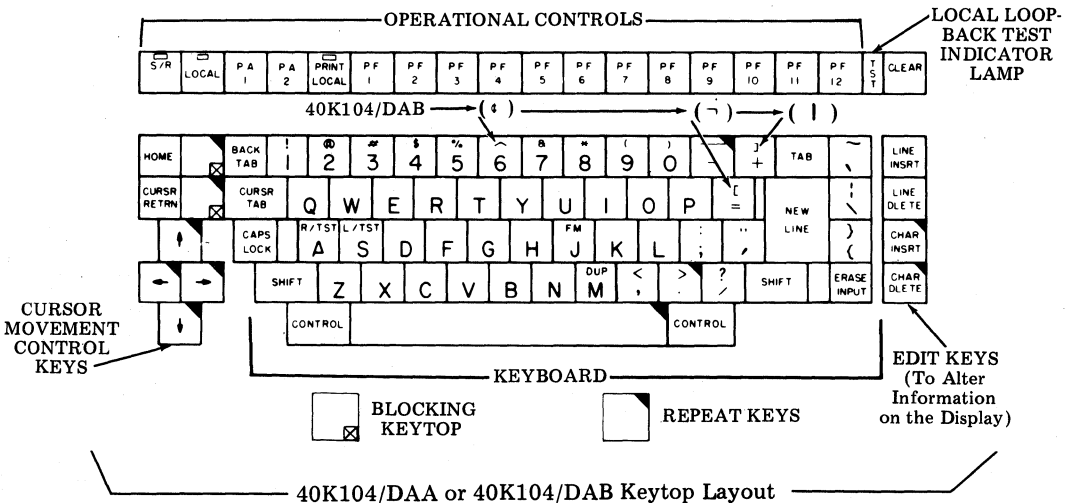
Fig. 5—Opcon Keypop Layouts
