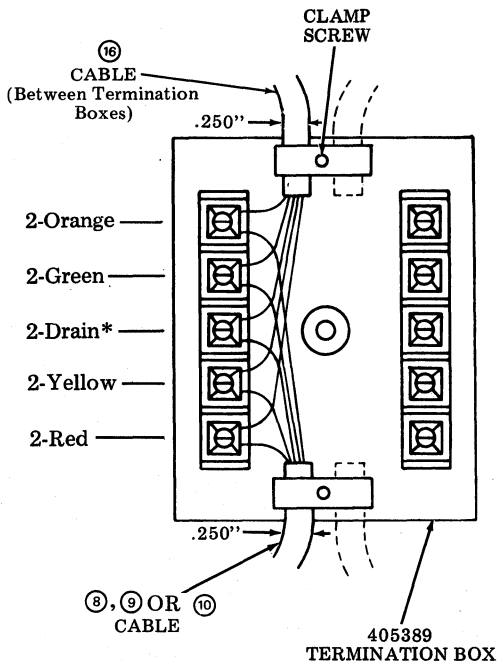
Fig. 15—405389 Termination Box ⑫ Wiring
