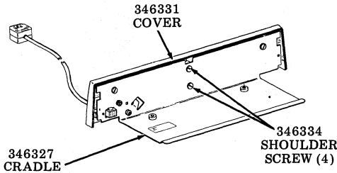
Fig. 5—40BSE201 Disassembly
