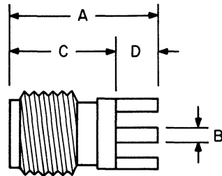
901-144 straight jack
