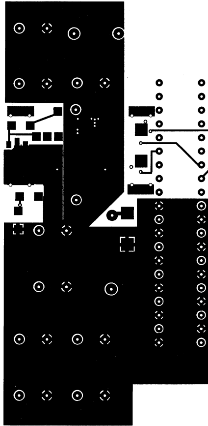
Bottom Layer
