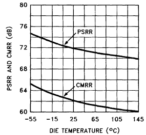
PSRR & CMRR vs Die Temperature
