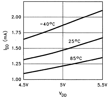
I DD vs V DD R SET = 681k
