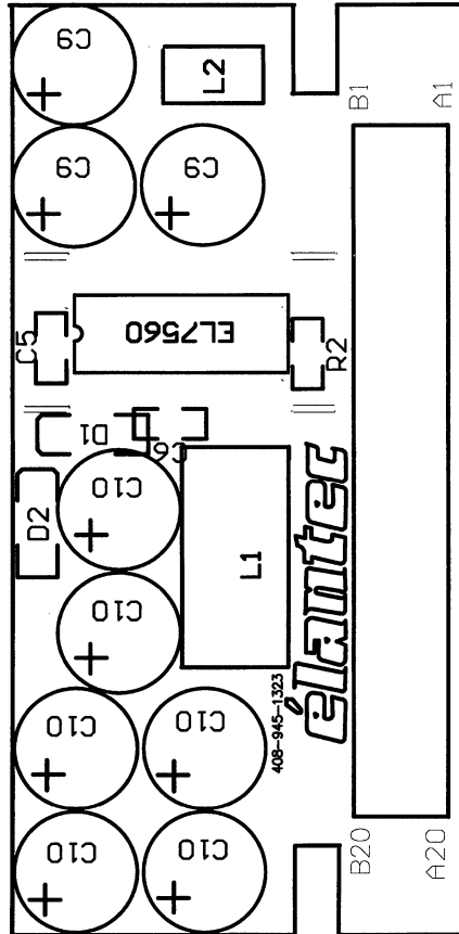
Top Layer Silkscreen
