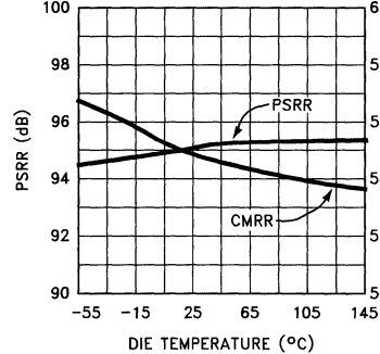
PSRR & CMRR vs Die Temperature
