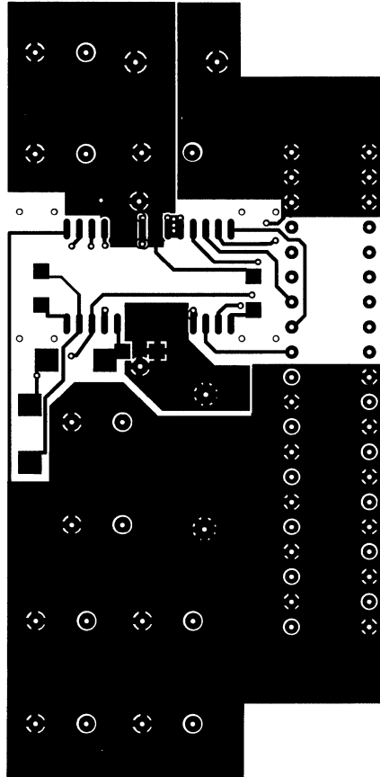
Top Layer
