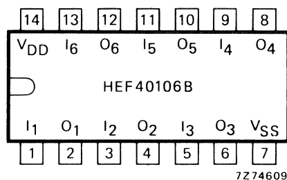
Fig. 2 Pinning diagram.
