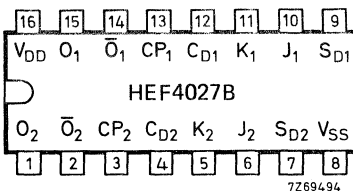
Fig. 2 Pinning diagram.
