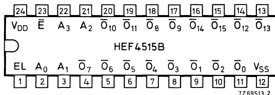
Fig. 2 Pinning diagram.
