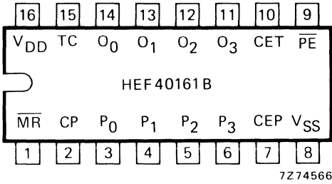
Fig. 3. Pinning diagram.
