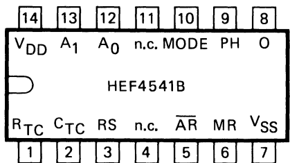
Fig. 2 Pinning diagram.
