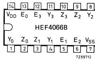
Fig. 2 Pinning diagram.
