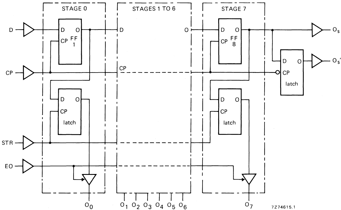
Fig. 3a Logic diagram.
