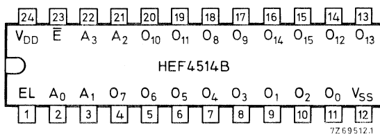
Fig. 2 Pinning diagram.
