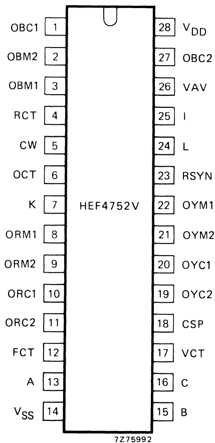
Fig. 1 Pinning diagram.
