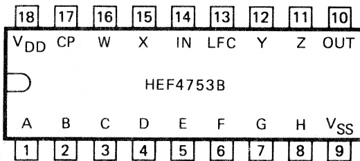
Fig. 2 Pinning diagram.
