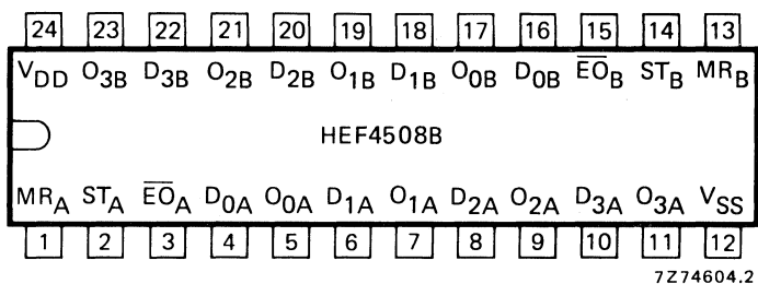
Fig. 2 Pinning diagram.
