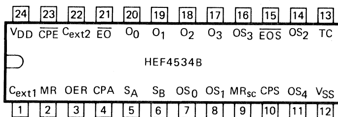
Fig. 1 Pinning diagram.
