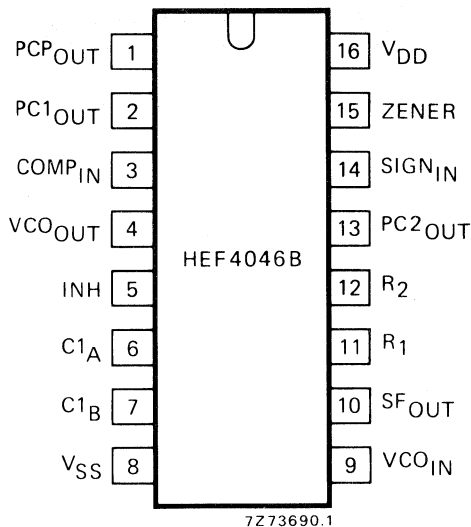
Fig. 2 Pinning diagram.
