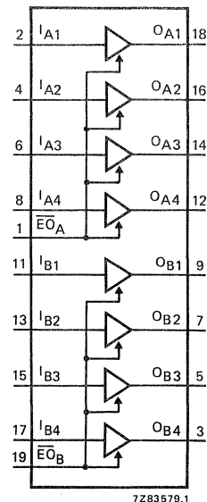
HEF40244B
