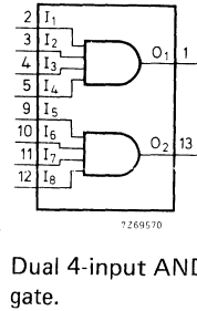
HEF4082B
