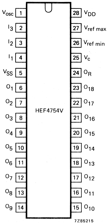
Fig. 2 Pinning diagram.
