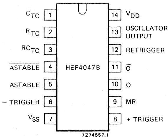
Fig. 2 Pinning diagram.
