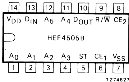
Fig. 1 Pinning diagram.
