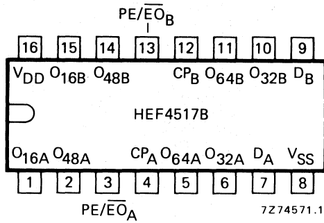
Fig. 2 Pinning diagram.
