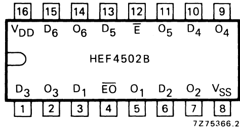
Fig. 2 Pinning diagram.
