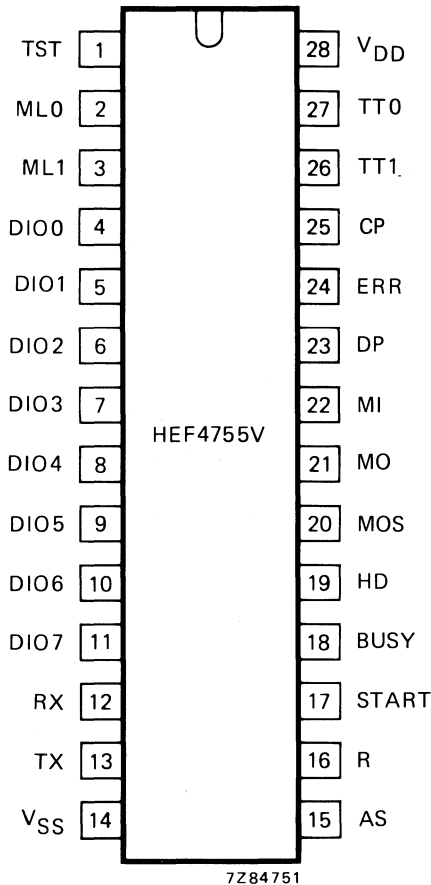
Fig. 1 Pinning diagram.
