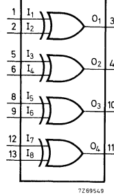
HEF4070B
