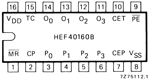
Fig. 3 Pinning diagram.
