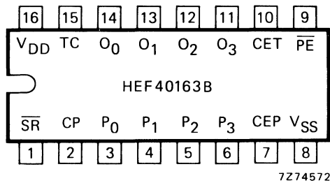
Fig. 3 Pinning diagram.
