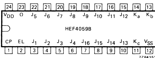
Fig. 2 Pinning diagram.
