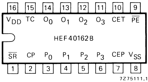
Fig. 3 Pinning diagram.
