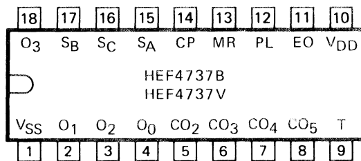
Fig. 1 Pinning diagram.
