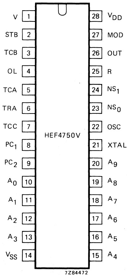
Fig. 1 Pinning diagram.
