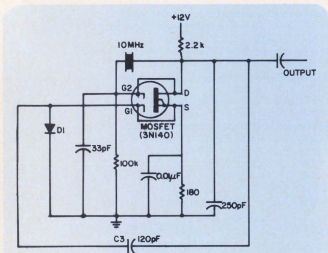
D1 - ANY GOOD SILICON RF DIODE
