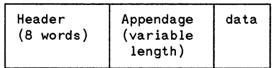
Figure 5-2. Basic DS message format (X.25). (not to scale)
